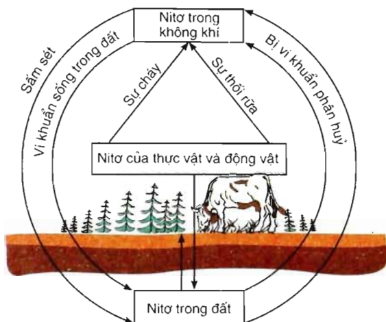
Hình 2.8. Chu trình của nitơ trong tự nhiên
