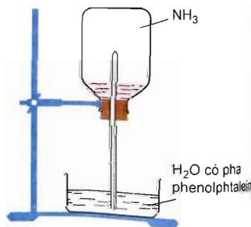
Hình 2.3. Sự hoà tan của amoniacc trong nước
