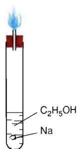
Hình 8.3. Đốt khí hidro sinh ra từ phản ứng của ethanol với natri
