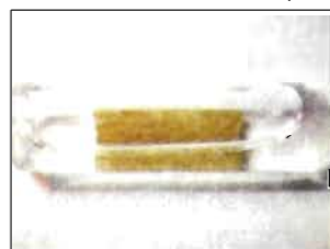
a) Photpho trắng
